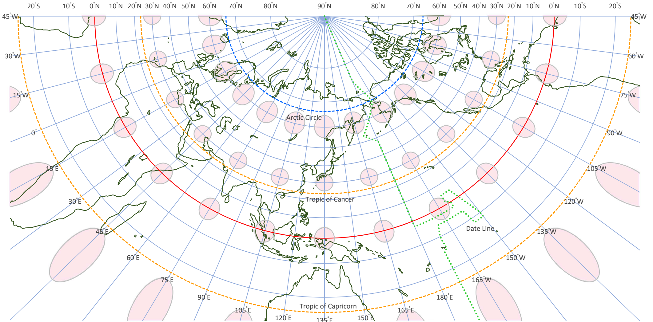
[図 9-5-3-5] Perspective Conic 図法 ( Perspective Conic Projection ) ティソーの指示楕円 ● 【地図主点(中心)】東経 135° 【標準緯度1】北緯20° 【標準緯度2】北緯40° 【経度間隔】15° 【緯度間隔】10°
