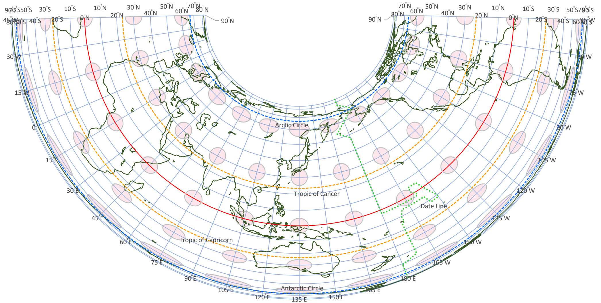
[図 9-5-3-2] アルベルス正積円錐図法 ( Albers Equal-area Conic Projection ) ティソーの指示楕円 ● 【地図主点(中心)】東経 135° 【標準緯度1】北緯20° 【標準緯度2】北緯40° 【経度間隔】15° 【緯度間隔】10°
