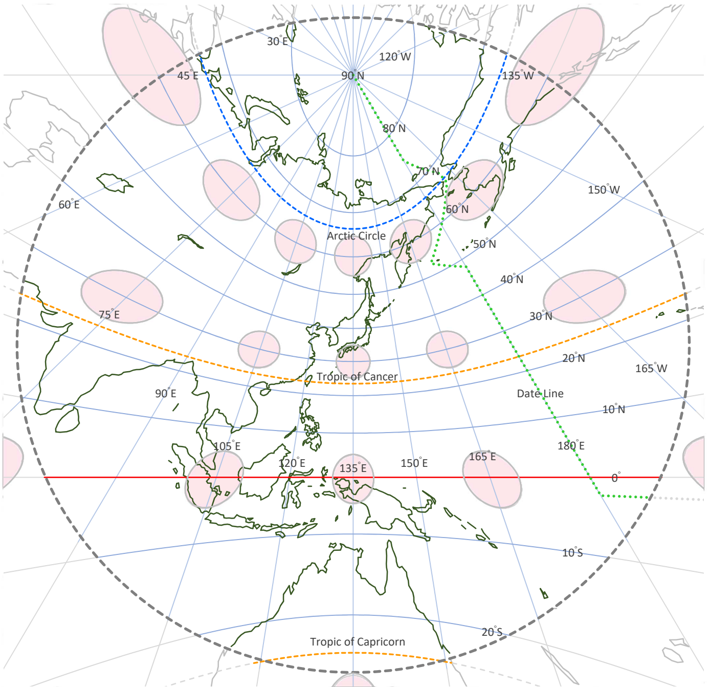
[図 9-5-5-1-3] 心射図法 - 傾斜面 ( Gnomonic Projection, Oblique Aspect )
