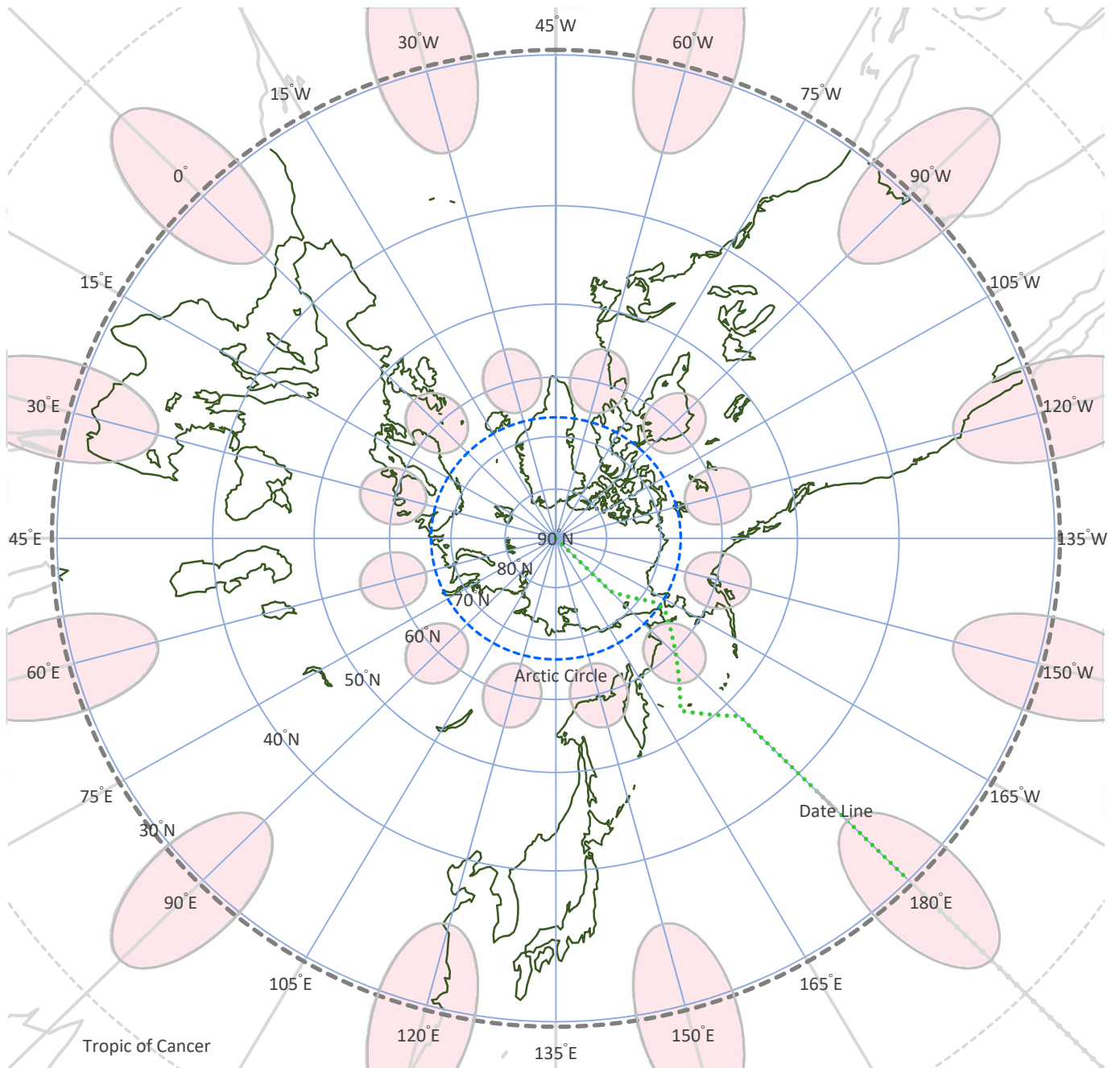
[図 9-5-5-1-1] 心射図法 - 極面 ( Gnomonic Projection, Polar Aspect ) ティソーの指示楕円 ●
