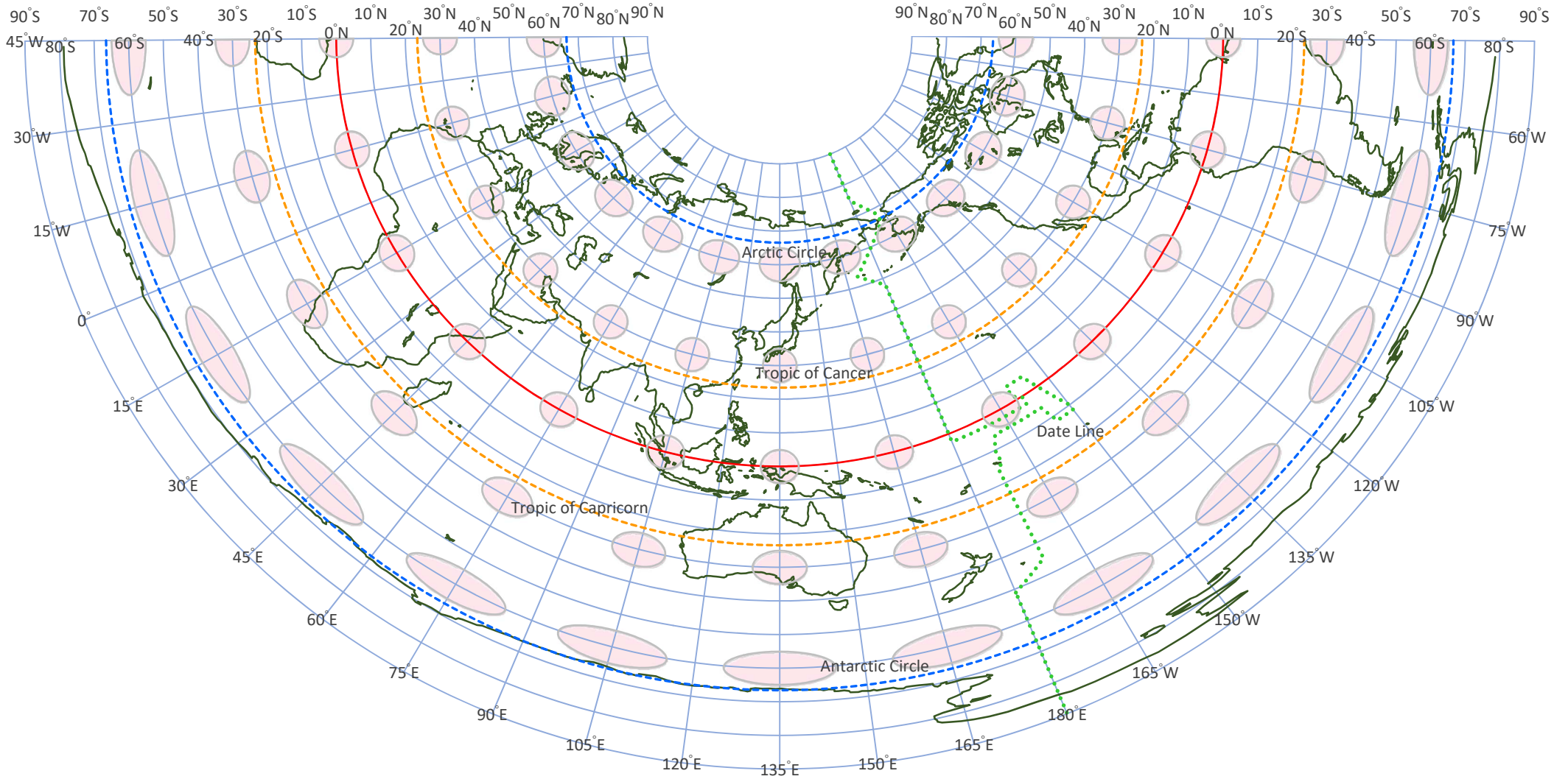
[図 9-5-3-1] 正距円錐図法 ( Equidistant Conic Projection ) ティソーの指示楕円 ● 【地図主点(中心)】東経 135° 【標準緯度1】北緯20° 【標準緯度2】北緯40° 【経度間隔】15° 【緯度間隔】10°
