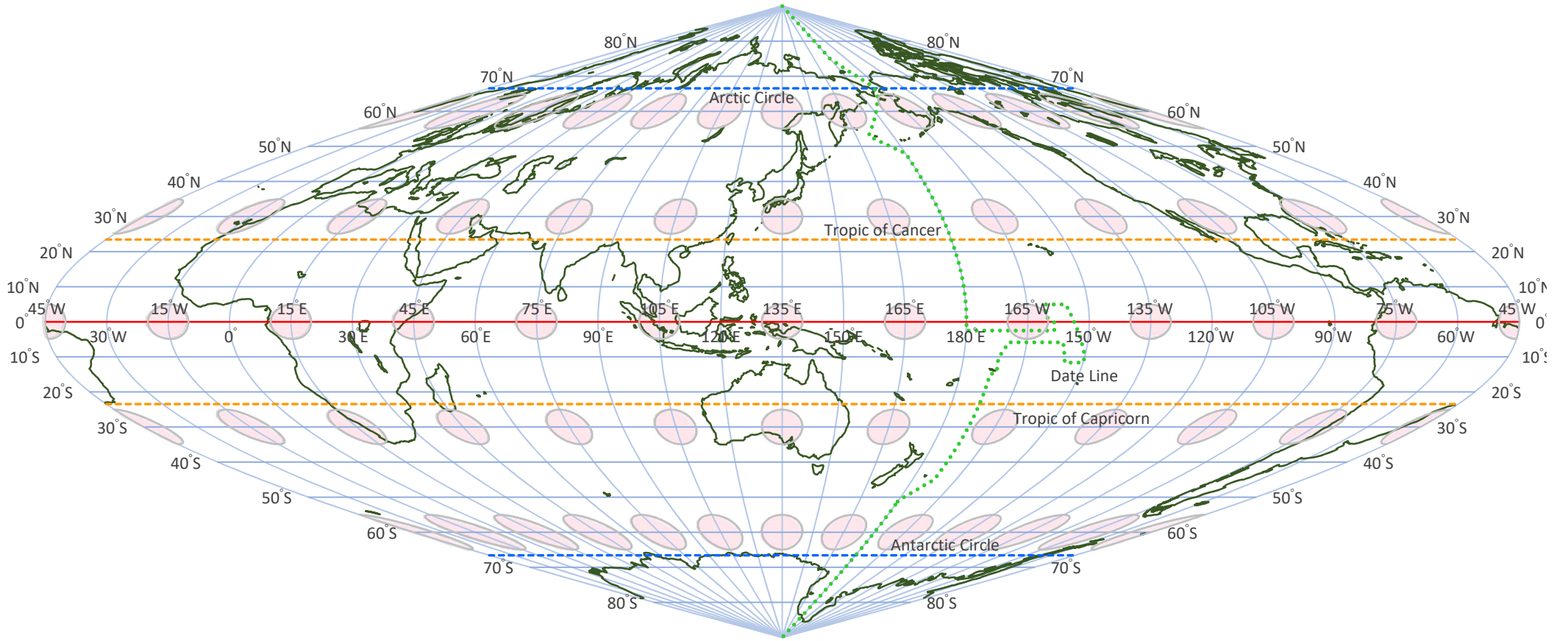
[図 9-5-2-1] サンソン図法 ( Sanson-Flamsteed Projection <Sinusoidal Projection>) ティソーの指示楕円 ● 【地図主点(中心)】 東経 135°、緯度 0° 【経度間隔】 15° 【緯度間隔】 10°
