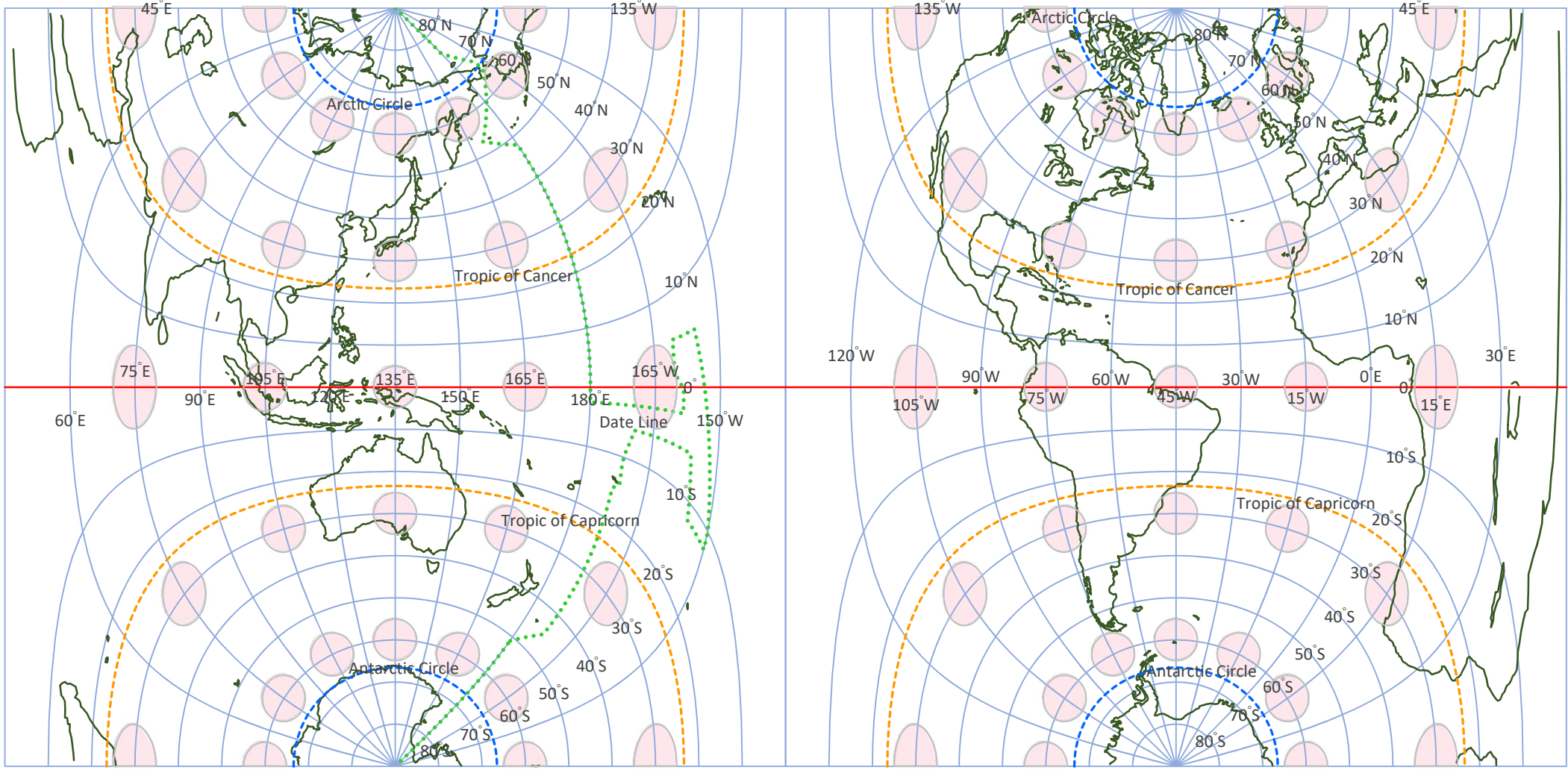
[図 9-5-1-4] カッシーニ図法 ( Cassini Projection ) ティソーの指示楕円 ● 【地図主点(中心)】西経 135°、緯度 0° 【経度間隔】15° 【緯度間隔】10°
