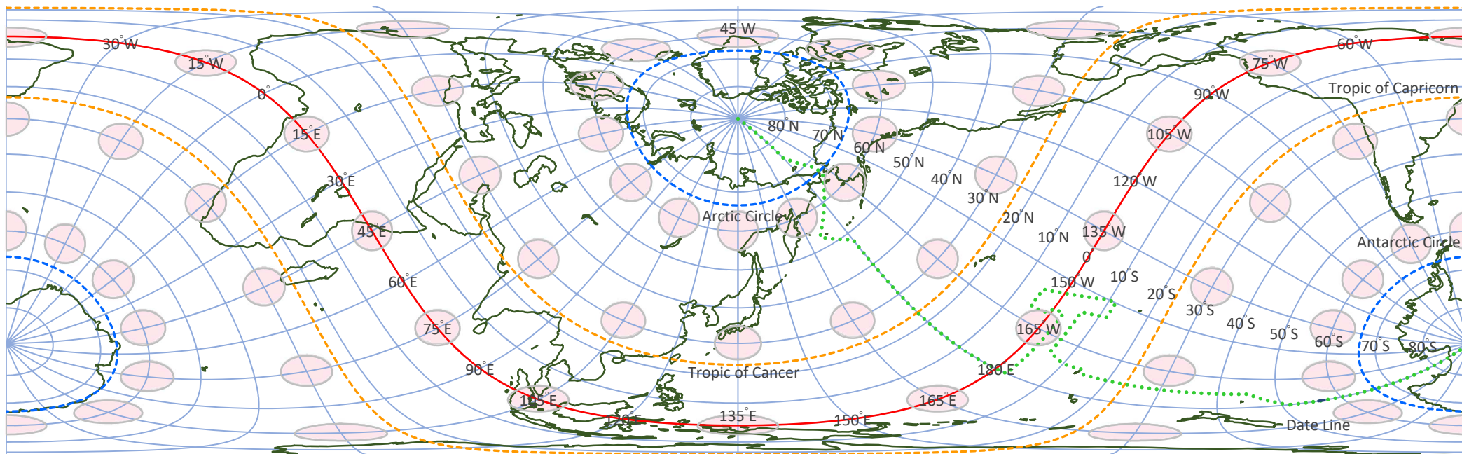
[図 9-5-1-3-3] 斜軸ランベルト正積円筒図法 ( Oblique Lambert Cylindrical Equal-Area Projection ) ティソーの指示楕円● 【傾斜経度緯度】西経 45°、北緯 30° 【経度間隔】15° 【緯度間隔】10°
