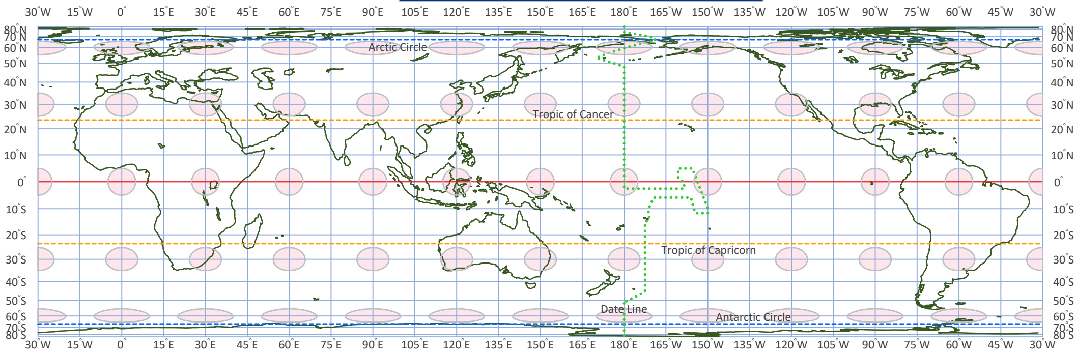
[図 9-5-1-3-1] ランベルト正積円筒図法 (Lambert Cylindrical Equal-Area Projection) ティソーの指示楕円●
