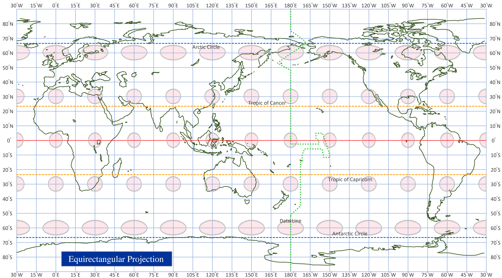
【図 9-5-1-2-2】 Equirectangular Projection ティソーの指示楕円● 【地図主点(中心)】 東経 150°、緯度 0° 【標準緯度】 30° 【経度間隔】 15° 【緯度間隔】 10°
