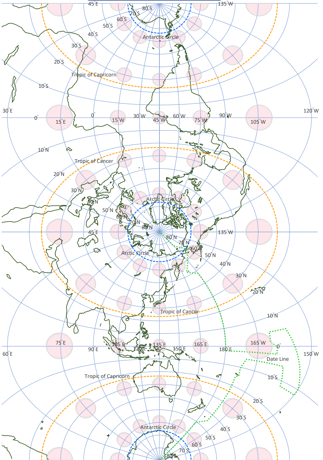
[図 9-5-1-1-2] 横軸メルカトル図法 ( Transverse Mercator Projection ) ティソーの指示楕円 ● 【地図主点(中心)】東経 135°、北緯 90° 【経度間隔】 15° 【緯度間隔】 10°
