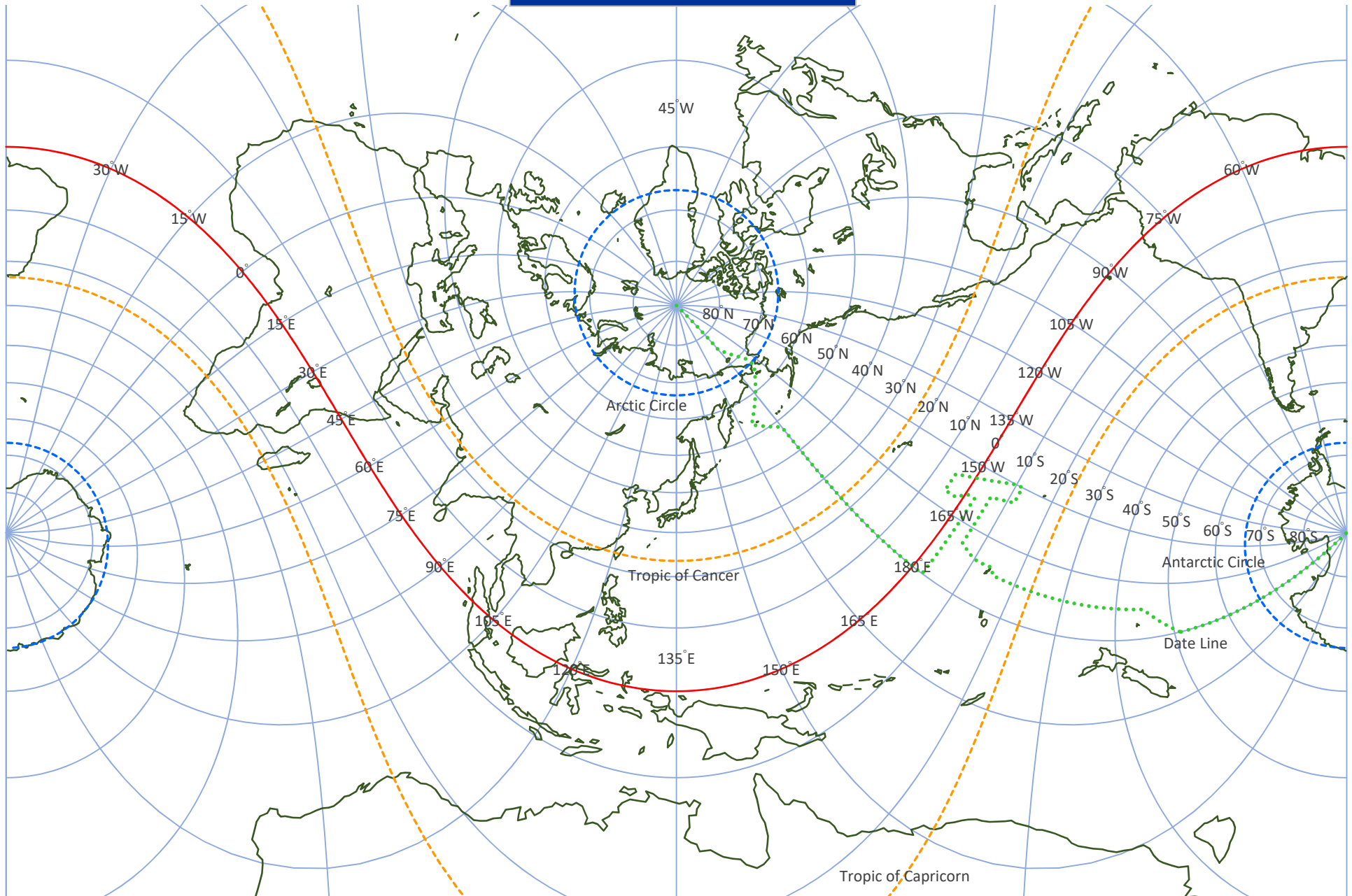
[図 6-1-4-1] 斜軸メルカトル図法 ( Oblique Mercator Projection )
