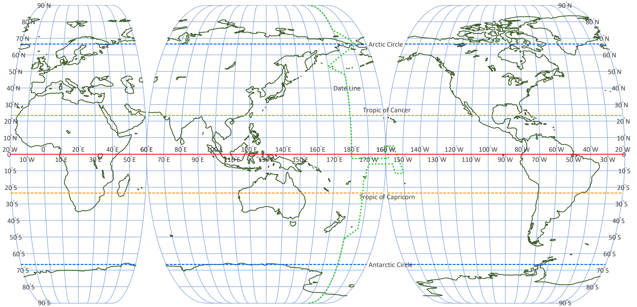
[図 7-2-3] 断裂エッケルト III 図法 ( Interrupted Eckert III Projection )
