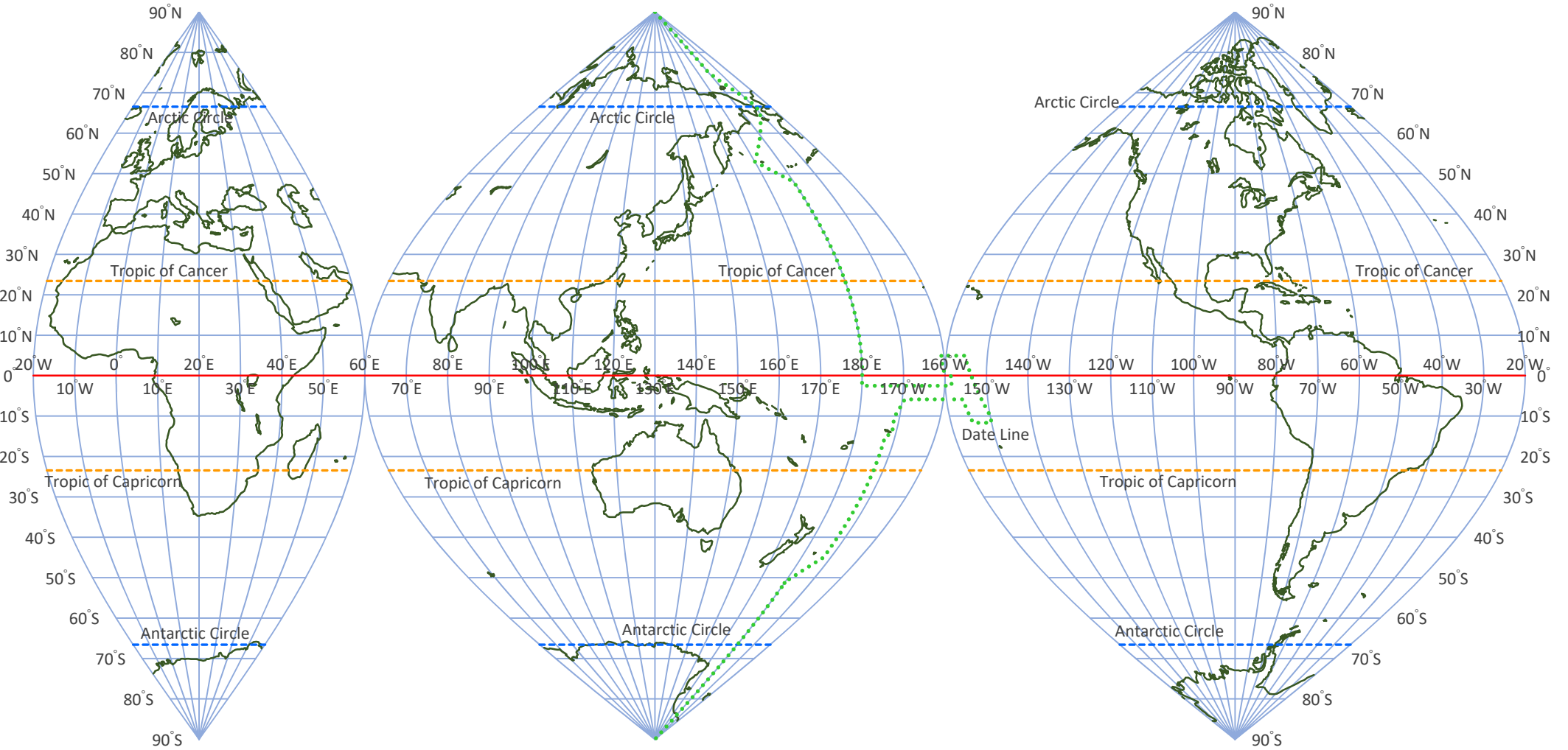
[図 7-2-1] 断裂サンソン図法 ( Interrupted Sinusoidal Projection )
