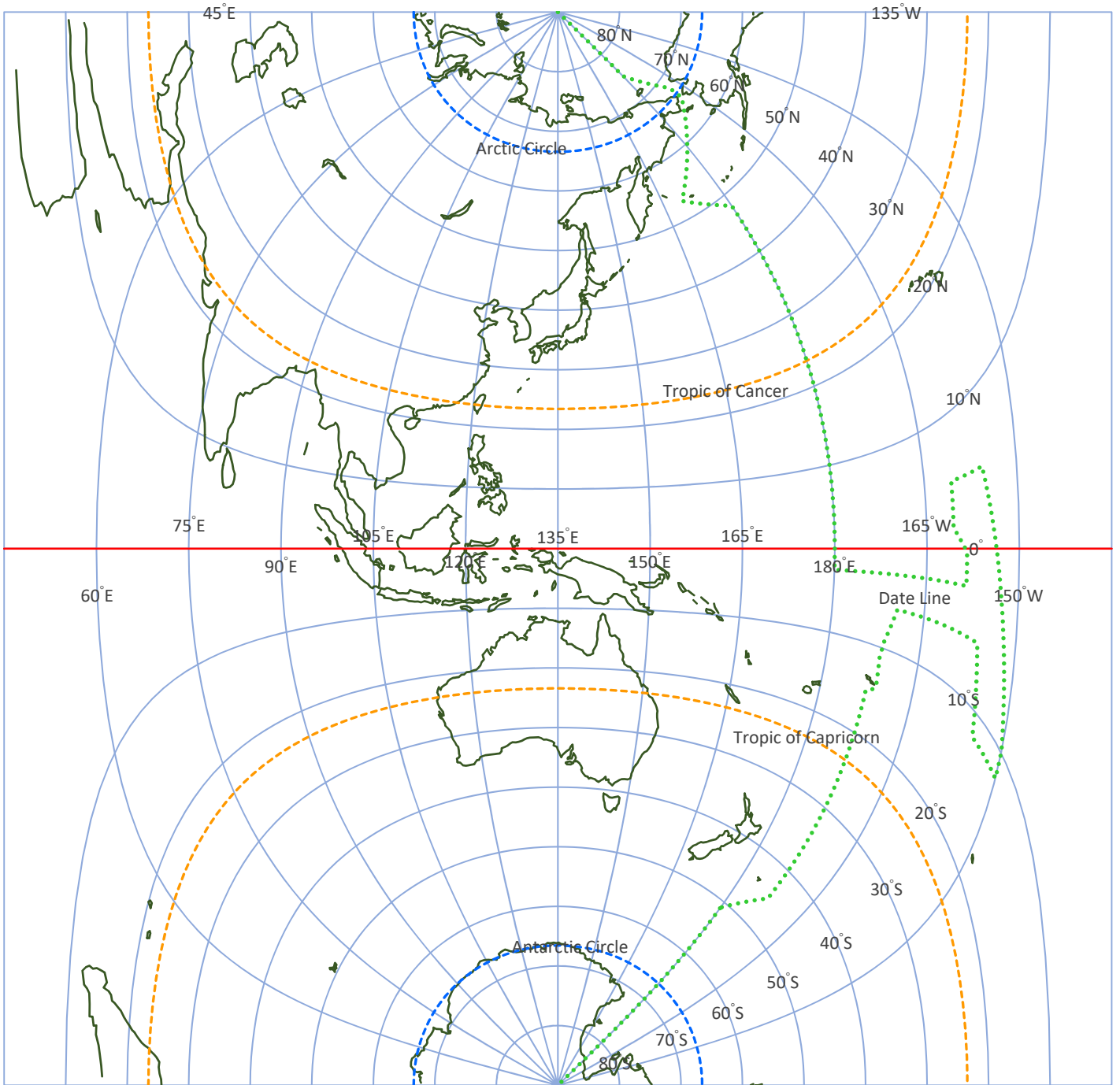
[図 6-1-3-4] カッシーニ図法 ( Cassini Projection ) 【地図主点(中心)】東経 135°、緯度 0° 【経度間隔】15° 【緯度間隔】10°
