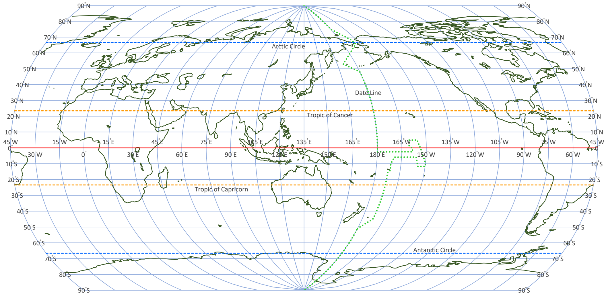
【図 6-7-1-3】 Apian I 図法 ( Apian I Projection )
