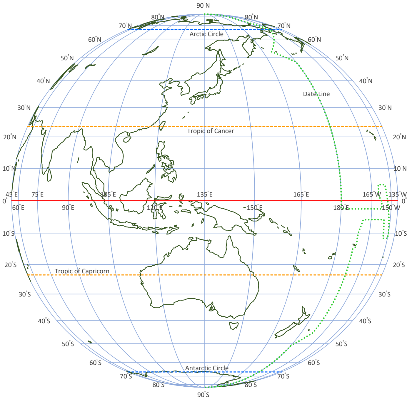
[図 6-5-1-4-2] 正射図法 - 赤道面 ( Orthographic Projection, Equatorial Aspect )
