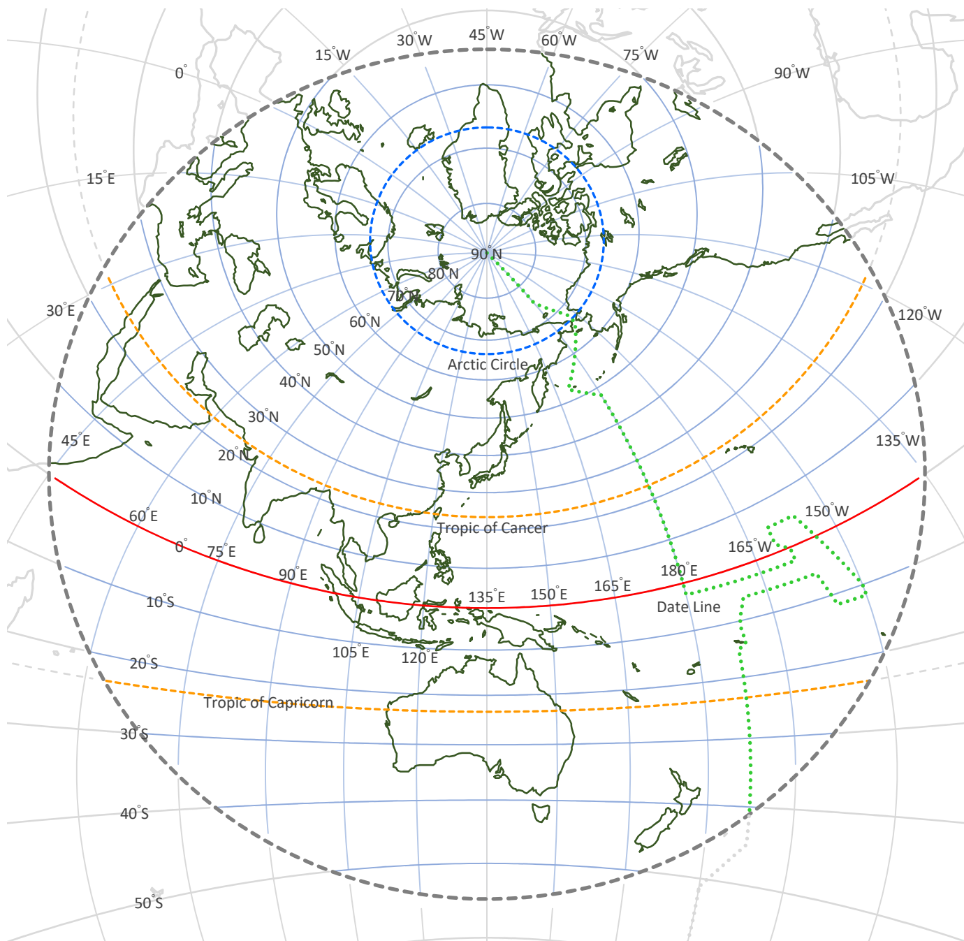
[図 6-5-1-2-3] 平射図法 - 傾斜面 ( Stereographic Projection, Oblique Aspect )
