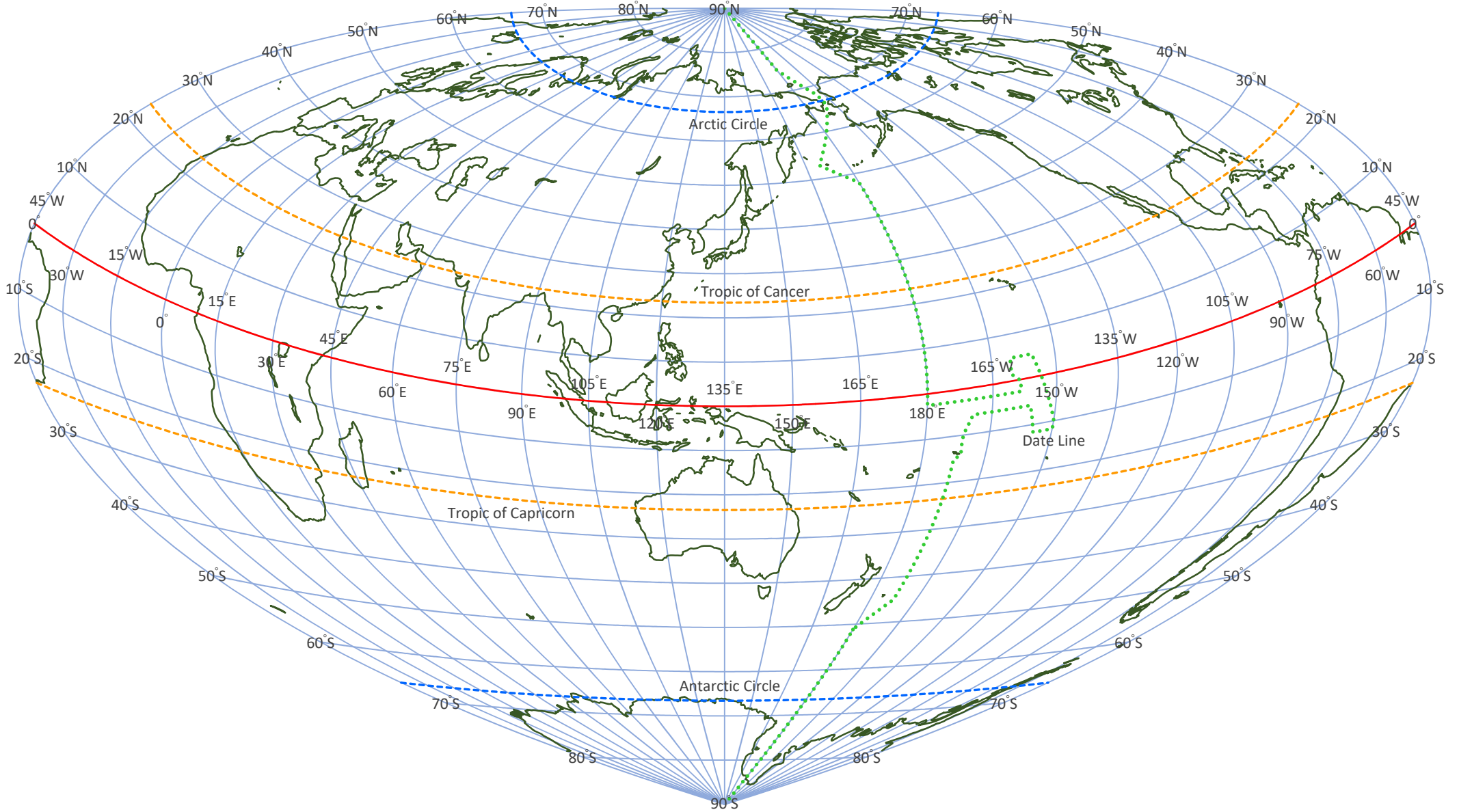
【図 6-4-3】 ボトムリー図法 ( Bottomley Projection )
