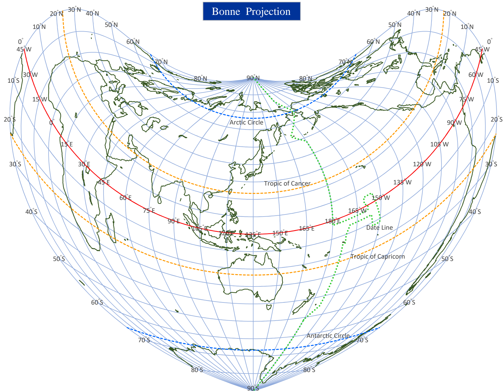
[図 6-4-1] ボンヌ図法 ( Bonne Projection )
