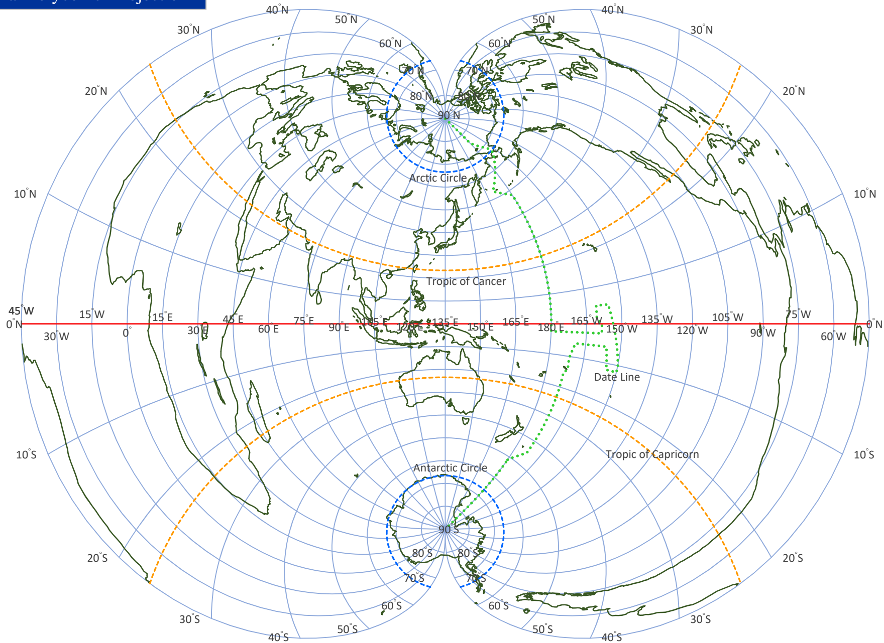
[图 6-3-6] 正規多圓錐圖法 ( Normal Polyconic Projection )
