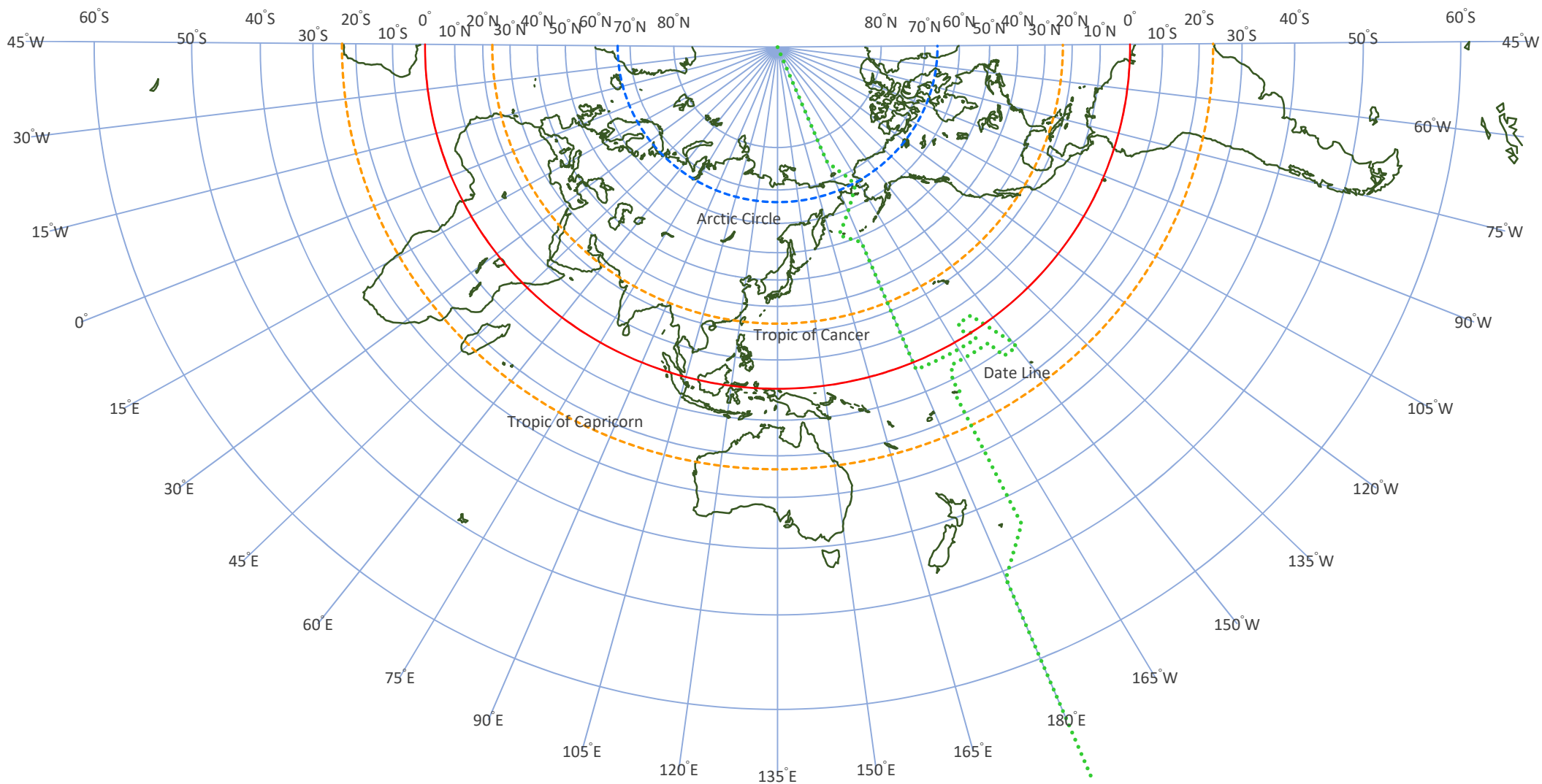
[図 6-3-4] ランベルト正角円錐図法 ( Lambert Conformal Conic Projection )
