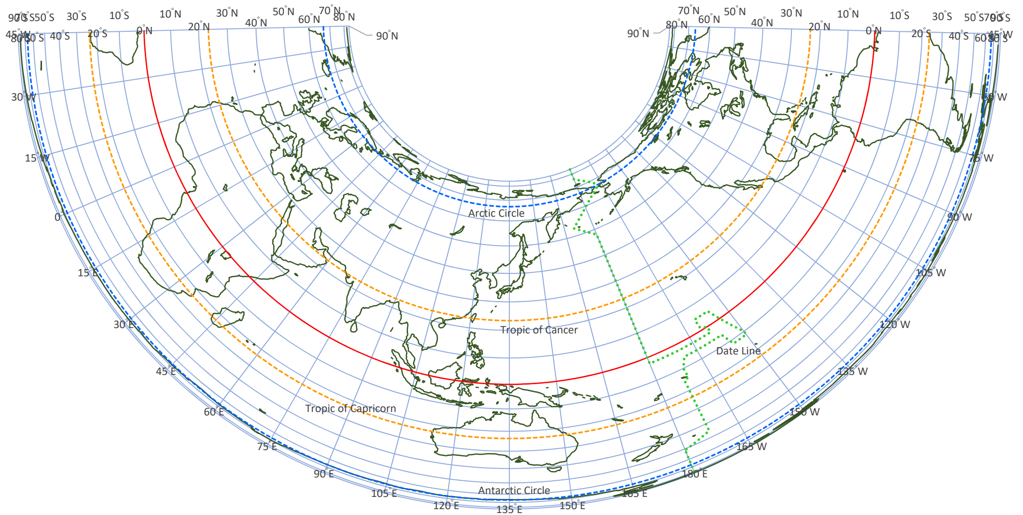
[図 6-3-2] アルベルス正積円錐図法 ( Albers Equal-area Conic Projection )
