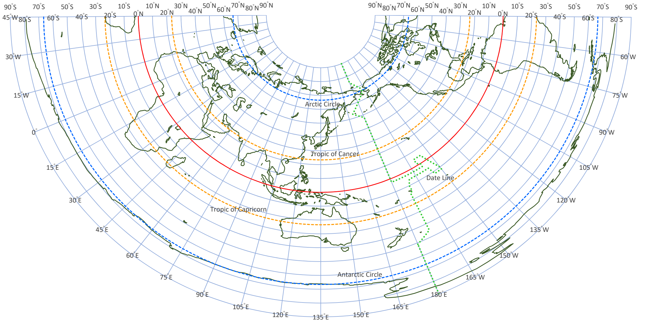
[图 6-3-1] 正距圆锥图法 ( Equidistant Conic Projection )
