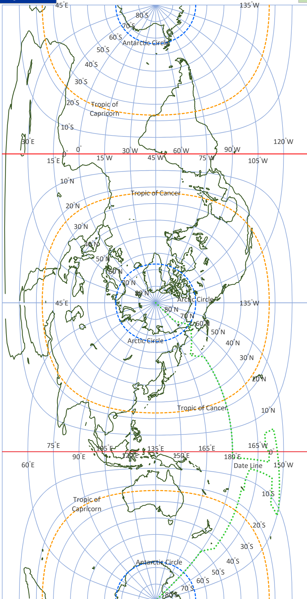
[図 6-1-3-4] カッシーニ図法 ( Cassini Projection )
