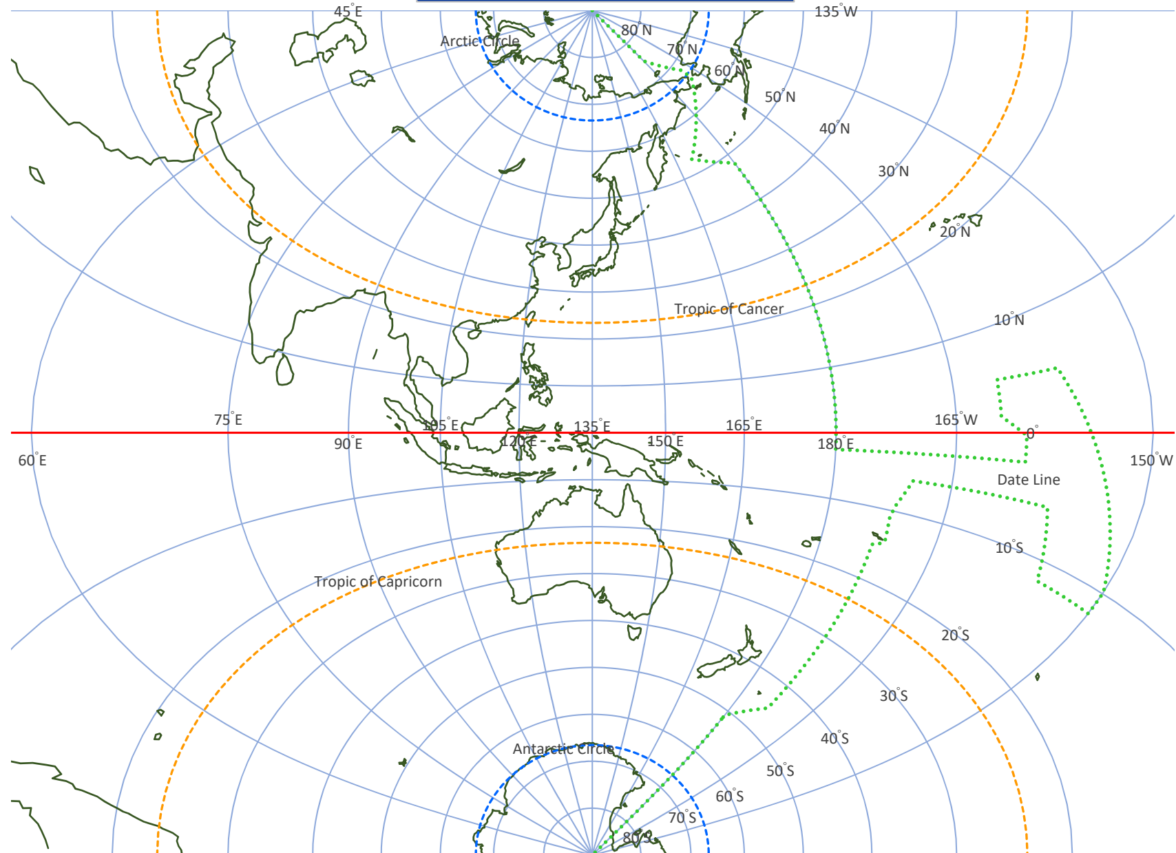
[図 6-1-3-1] 横軸メルカトル図法 ( Transverse Mercator Projection )
