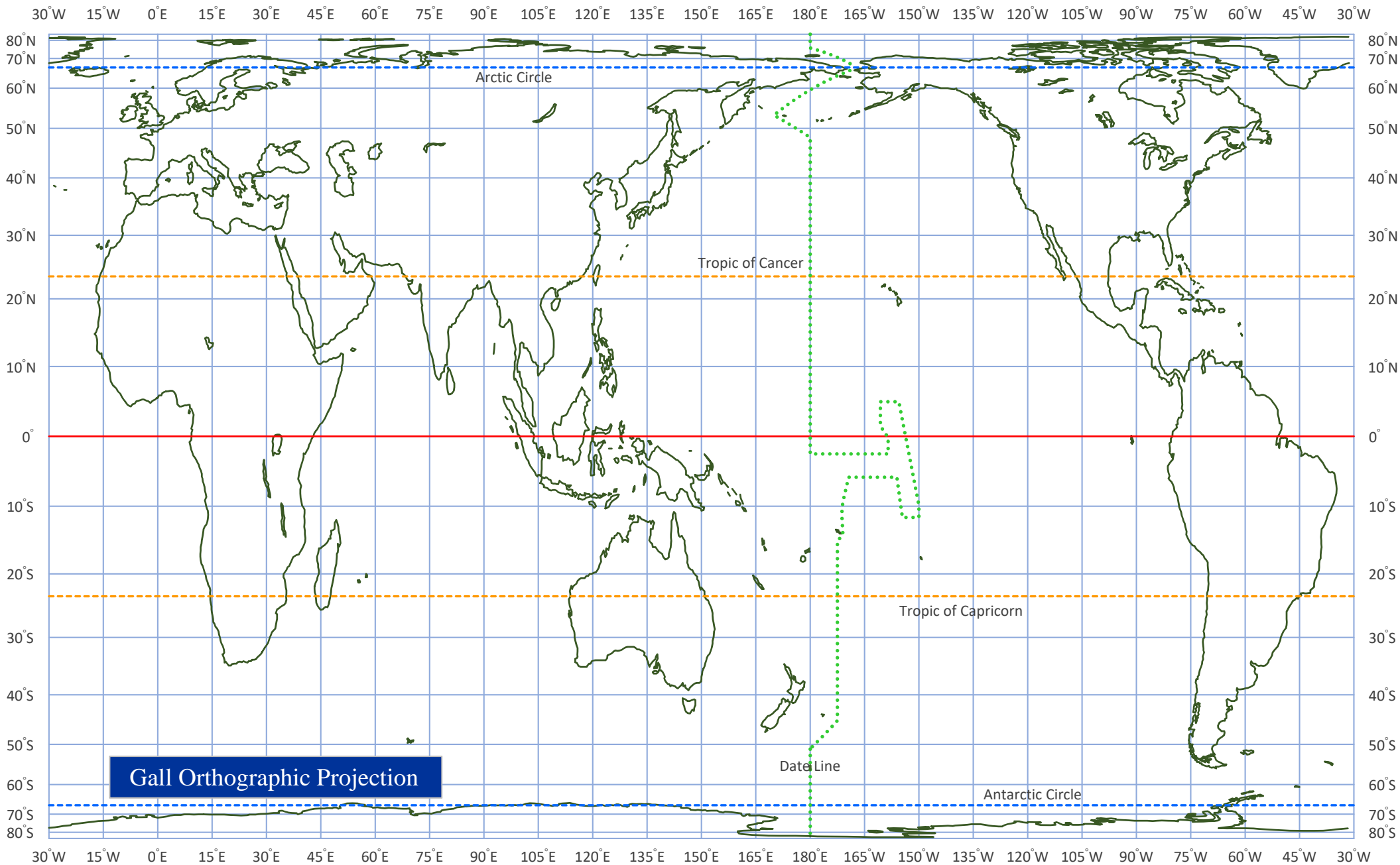
【図 6-1-2-6】 ゴール正射図法 ( Gall Orthographic Projection ) 【地図主点(中心)】 東経 150°、緯度 0° 【標準緯度】 45° 【経度間隔】 15° 【緯度間隔】 10°
