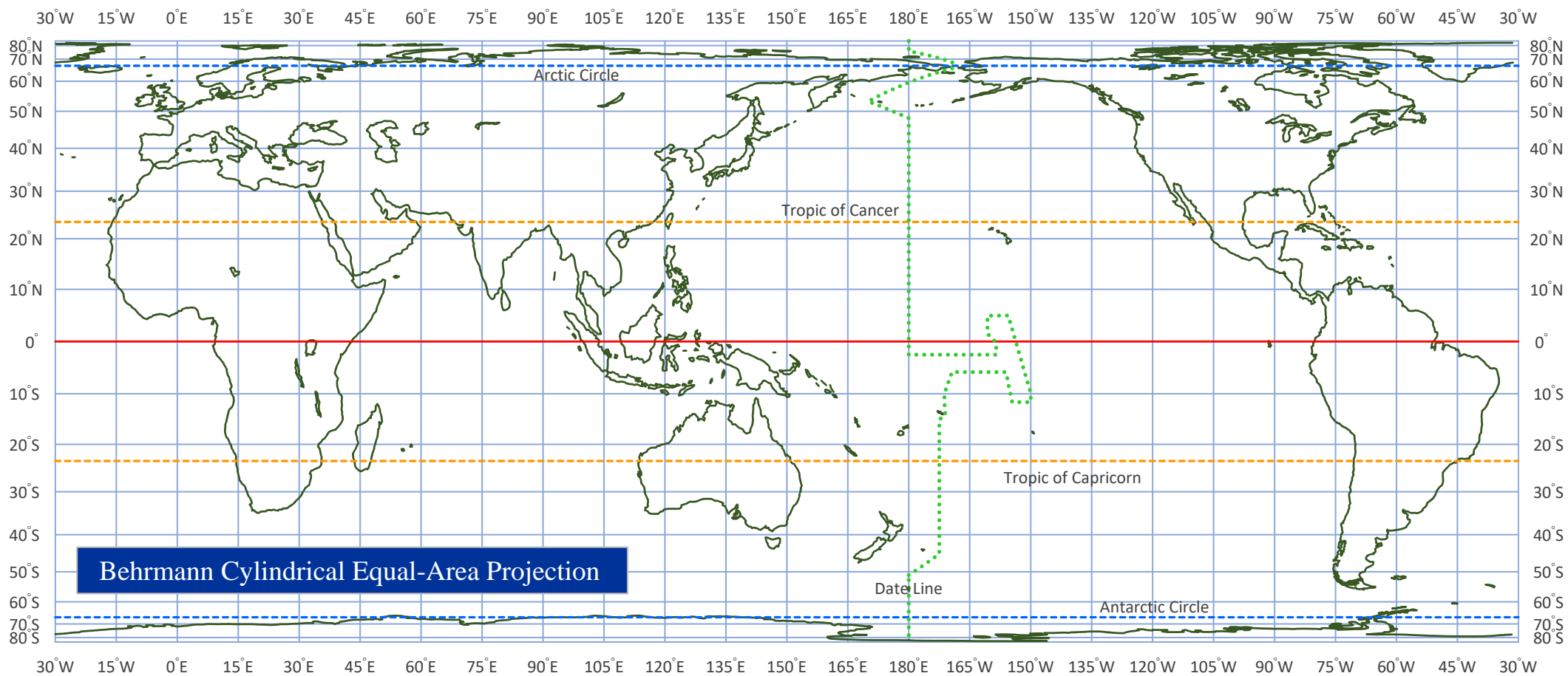
[図 6-1-2-1] ベールマン図法 ( Behrmann Cylindrical Equal-Area Projection )
