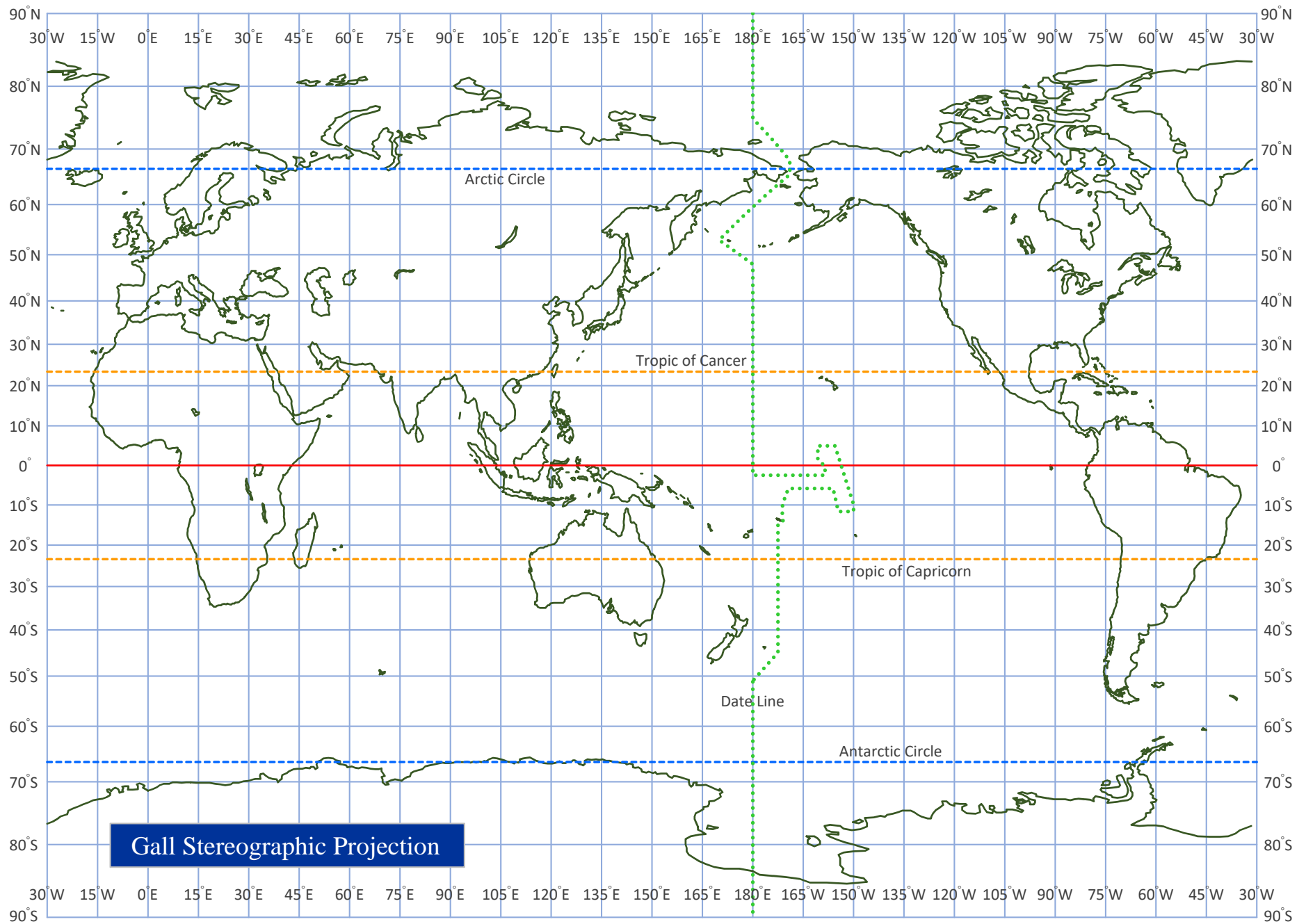
【図 6-1-1-7】 ゴール平射図法 ( Gall Stereographic Projection )
