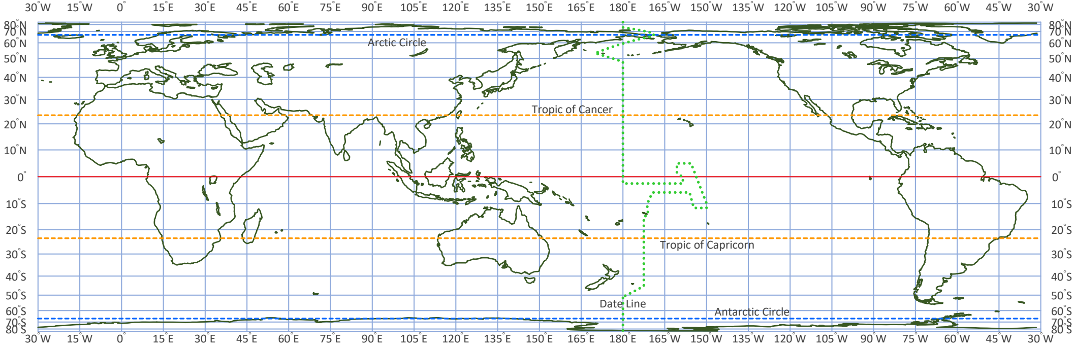
[図 6-1-1-4] ランベルト正積円筒図法 ( Lambert Cylindrical Equal-Area Projection )
