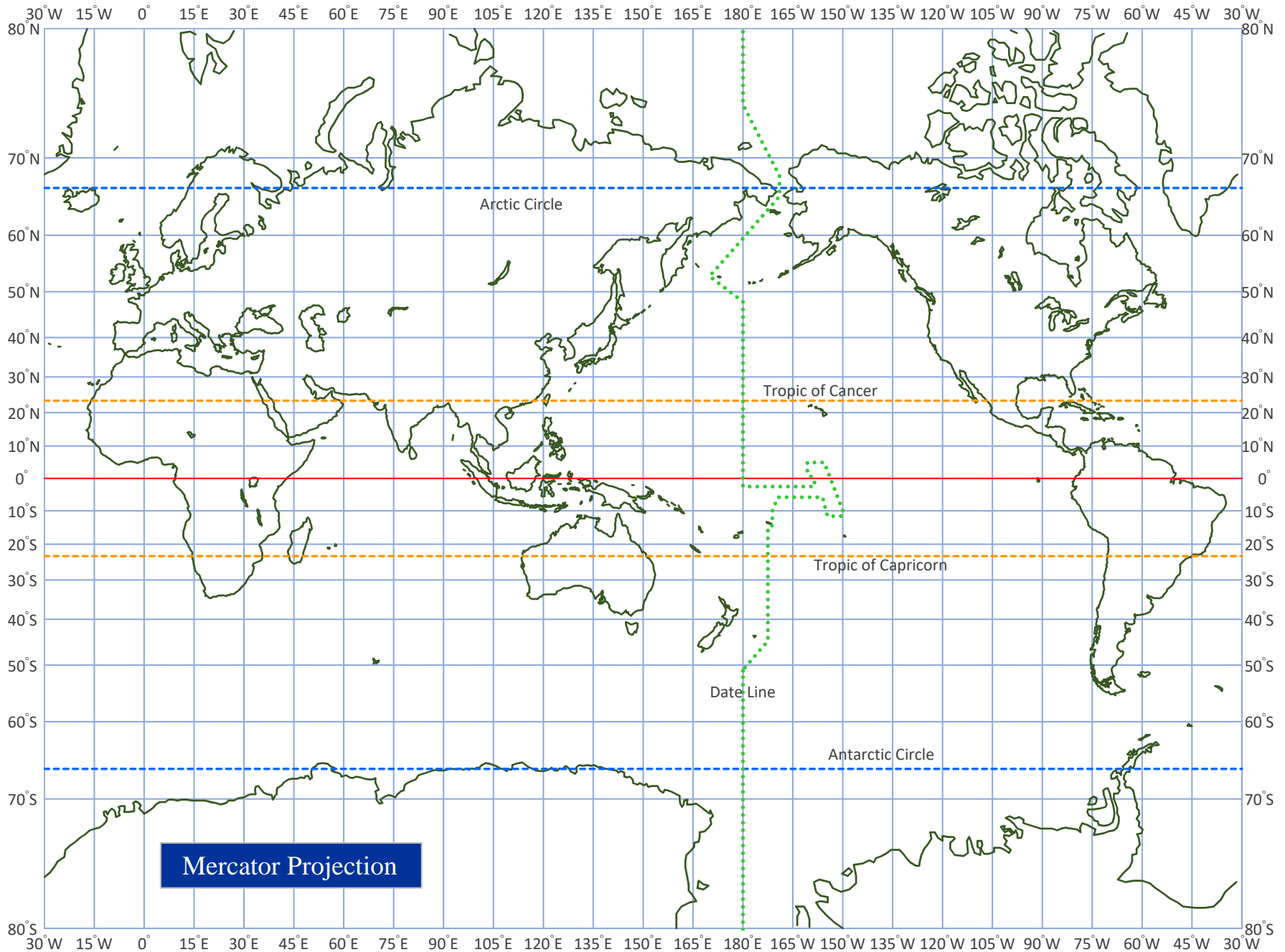
[図 6-1-1-1] メルカトル図法 ( Mercator Projection )
